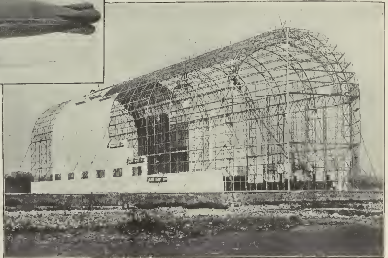
Cobertizo que actualmente se construye en Issy-les-Moulineaux para el globo dirigible «Clement-Bayard» En Inglaterra se construirá uno igual que costará 125.000 francos (De fotografía de World's Graphic Press.)
